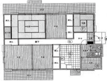
建屋平面図
